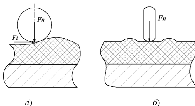
Рисунок 1 – Сдвиг дорожного покрытия под действием сил со стороны колеса автомобиля: а – на участках торможения образуются поперечные волны; б – на перегонах образуется остаточная деформация в виде колеи
