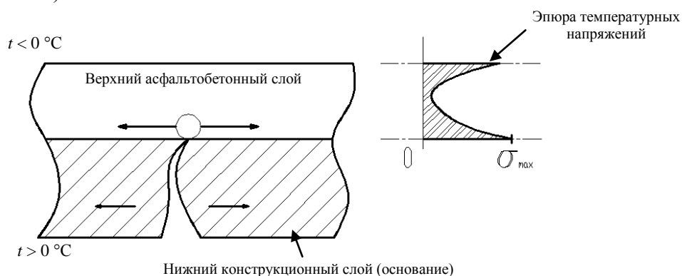
Рисунок 2 – Напряжения в асфальтобетонном слое покрытия, вызванные суточными колебаниями температуры
