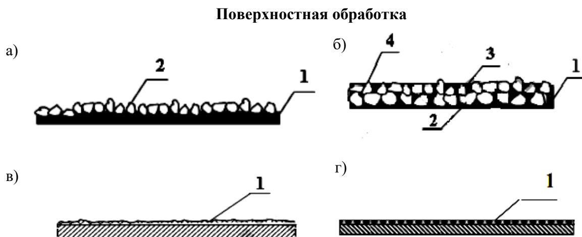
Рисунок 1 – Конструкции защитных слоев:
