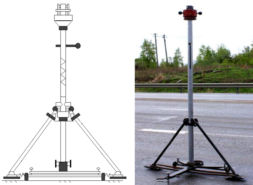
Рисунок 4 – Портативный прибор ППК для измерения коэффициента сцепления
