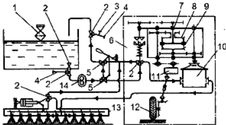
Рисунок 2 – Дозировочно-распределительная система автогудронатора: 1 – люк цистерны; 2 – кран; 3 – штуцер; 4 – трубопроводы для выдачи и приема вяжущего; 5 – циркуляционный кран; 6 – система ОПР; 7 – выходной вал; 8 – солнечная шестерня; 9 – ось сателлитов; 10 – расходомер; 11 – вариатор; 12 – опорное колесо; 13 – распределительная рампа; 14 – битумный насос для перекачки вяжущего
